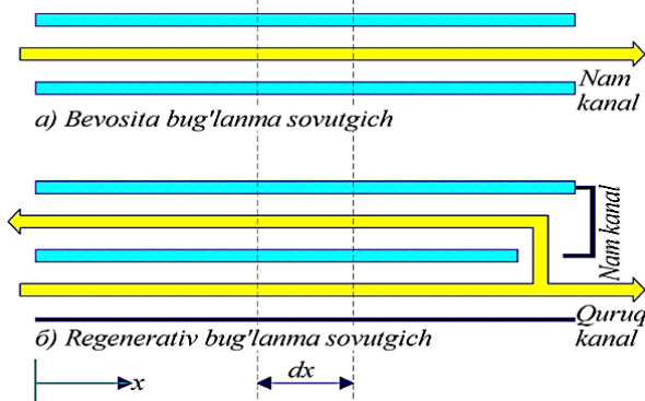
3-rasm. Bevosita bilvosita rejimli issiqlik va massa almashtirgich sxemasi
